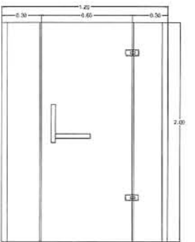
ALZADO
